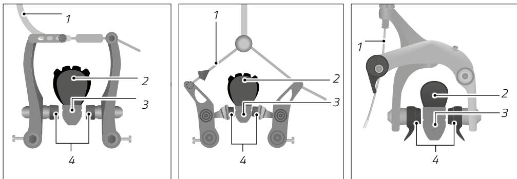
Sl.: Mehanske zavore na obroču (na podlagi primera)
