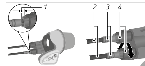
Sl.: Zračnost ohišja prestavnega potezala (levo) in nastavitveni vijak (desno) (na podlagi primera)
