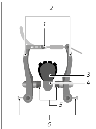
Sl.: Zavora na obroču s poteznim vodom (na podlagi primera)
