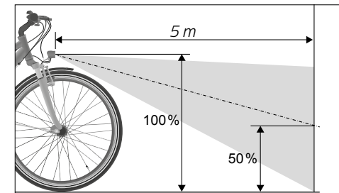
Sl.: Nastavitev žarometa (na podlagi primera)
