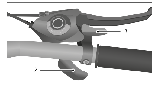
Sl.: Upravljalna enota na volanu za preklapljanje pastorkov in verižnih listov (tukaj na podlagi primera na desnem volanu)
