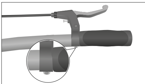
Sl.: Položaj zavorne ročice (na podlagi primera)
