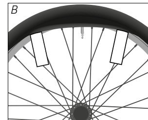
Sl.: Demontaža žičnatih ali nagubanih plaščev (na podlagi primera)
